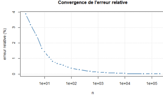
FIGURE 2 – Erreur relative \|\text{cov}_{emp}(n) - C^*\|/\|C^*\| en fonction de n
